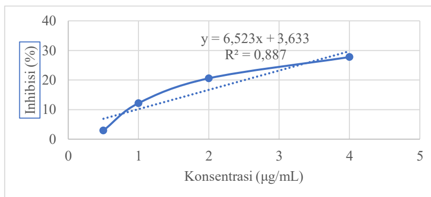
Gambar 5 Grafik Persamaan Regresi Linear Antioksidan Vitamin C
