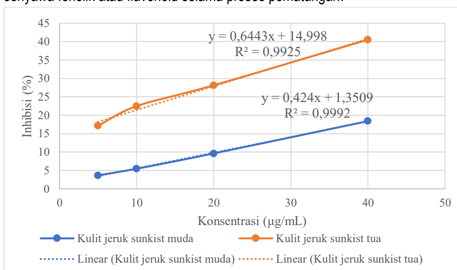
Gambar 4 Grafik Persamaan Regresi Linear Aktivitas Antioksidan Ekstrak Kulit Jeruk Sunkist Muda dan Tua
