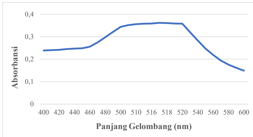
Gambar 1 Grafik Panjang Gelombang Serapan Maksimum DPPH
